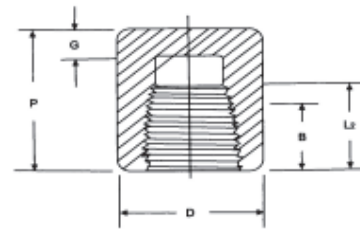
Cap
